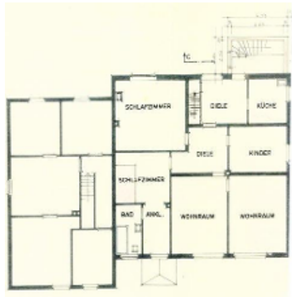
Grundriss OG beide Wohnungen
