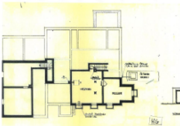
Grundriss KG
