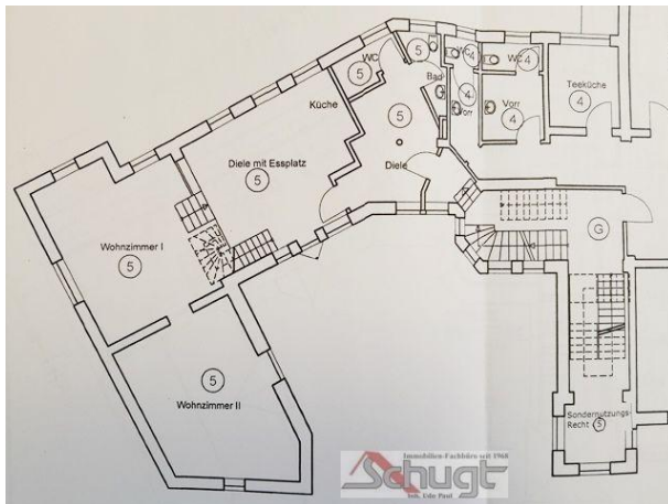
Grundriss 1. OG
