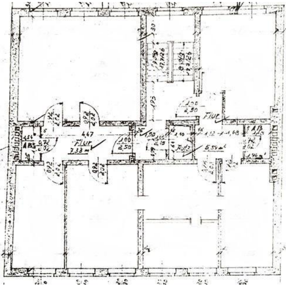
Grundriss
